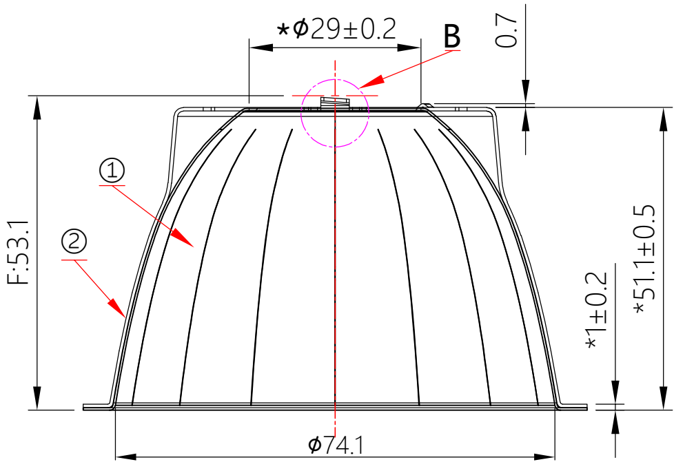
A-A
